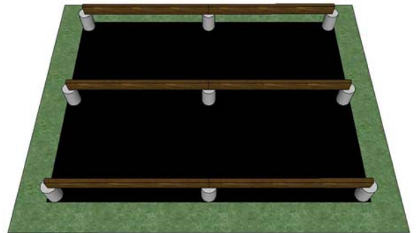
Poutres porteuses 160X50 mm longueur 3m
