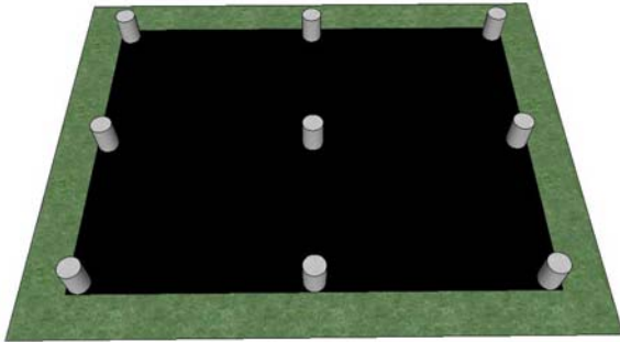
Pose de Bidim (évite les repousses d'herbes)
